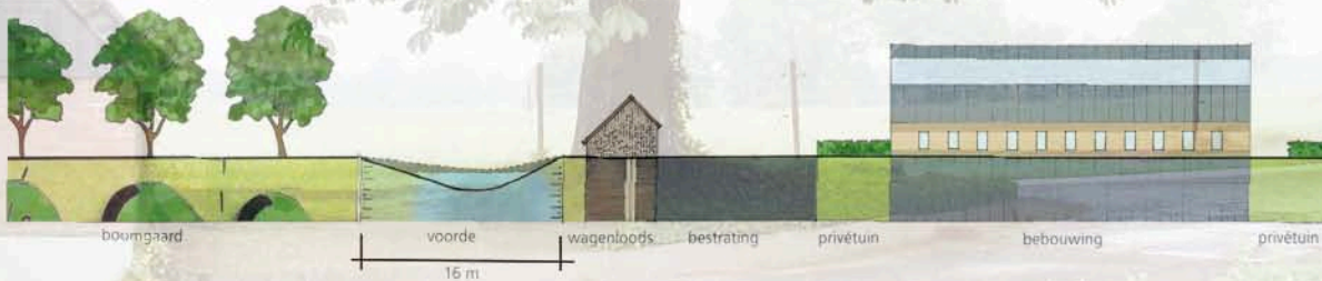
Doorsnede DD boomgaard, watergang en achtererf
