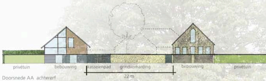
Doorsnede AA achtererf
